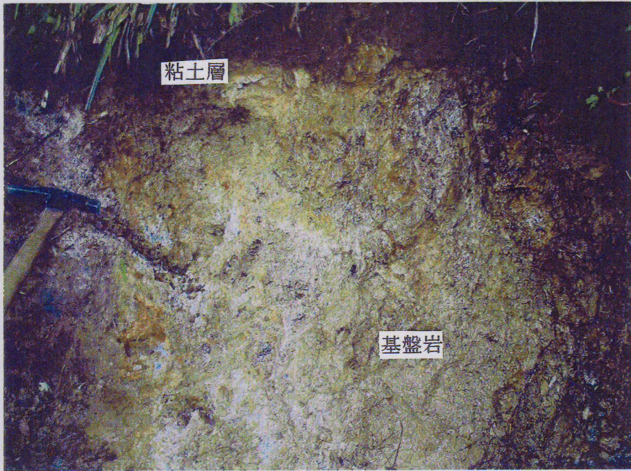
図-4-20 ⑦の地すべりの基盤と下底粘土層：粘土層の上から湧水あり
