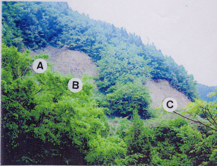
図-4-14 ⑥の地すべりの全体の露頭写真
