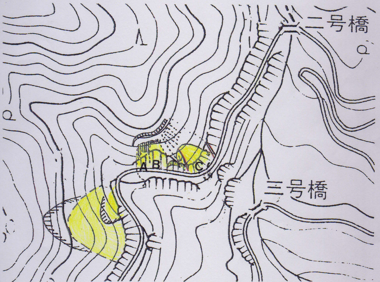
図-4-13 ⑥の地すべりの全体の地形区分 ㉑: 滑落崖
