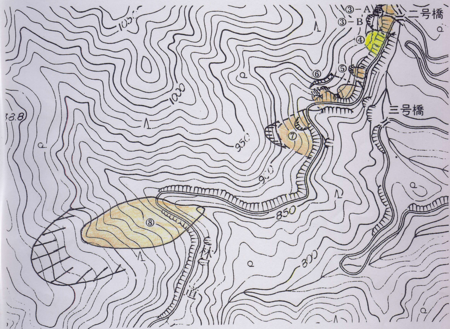
図-4-4 二号橋より南側約800m区間において空中写真判読と地表踏査 によって明らかにされた地すべり地形と初期の変形地形
