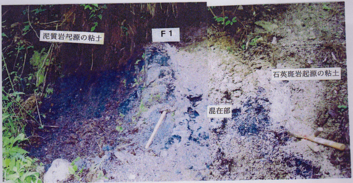
図-2-3 F1断層の露頭
