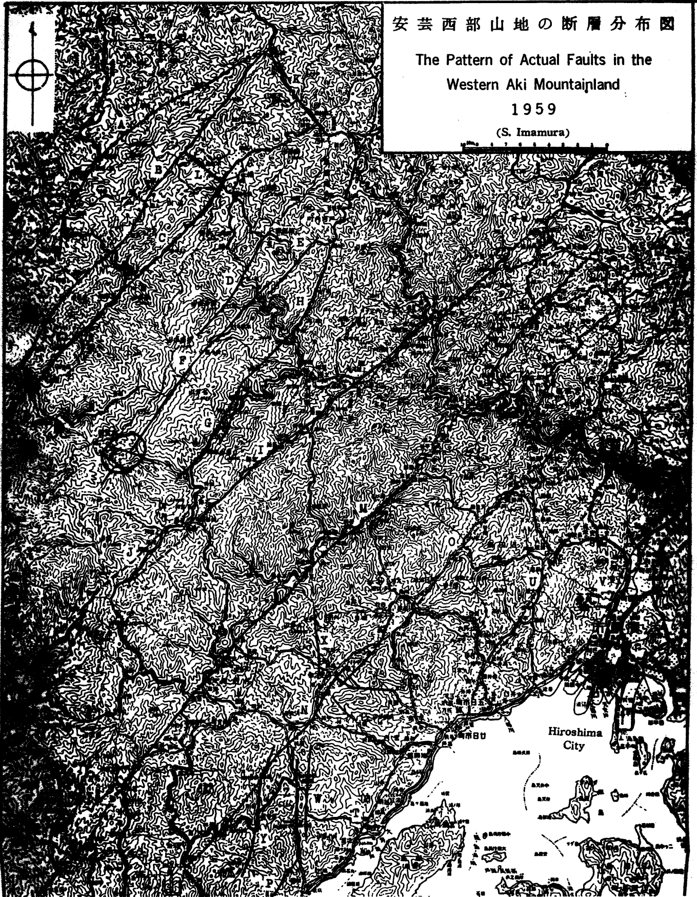
図-1-1 細見谷地域とその周辺に発達するNE-SW系断層群 (今村ほか、1959を一部改変：○内は調査地域)
